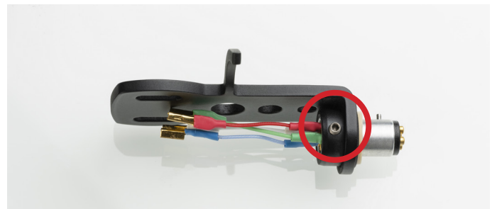
Inklusive Azimut-Einstellschraube
