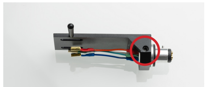
Einteiliges CNC-gefrästes Aluminium inklusive Azimut-Einstellschraube
